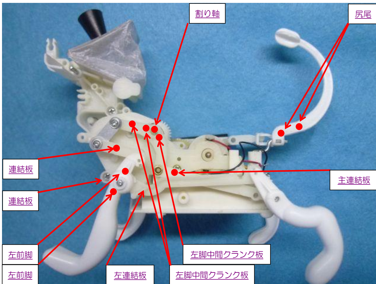
(2) 左側面
