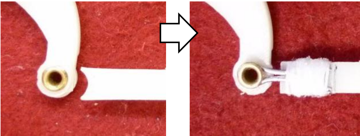
例5 修復前 ⇒ ステンレス線φ0.3+φ0.9+縫製糸+瞬間接着剤
