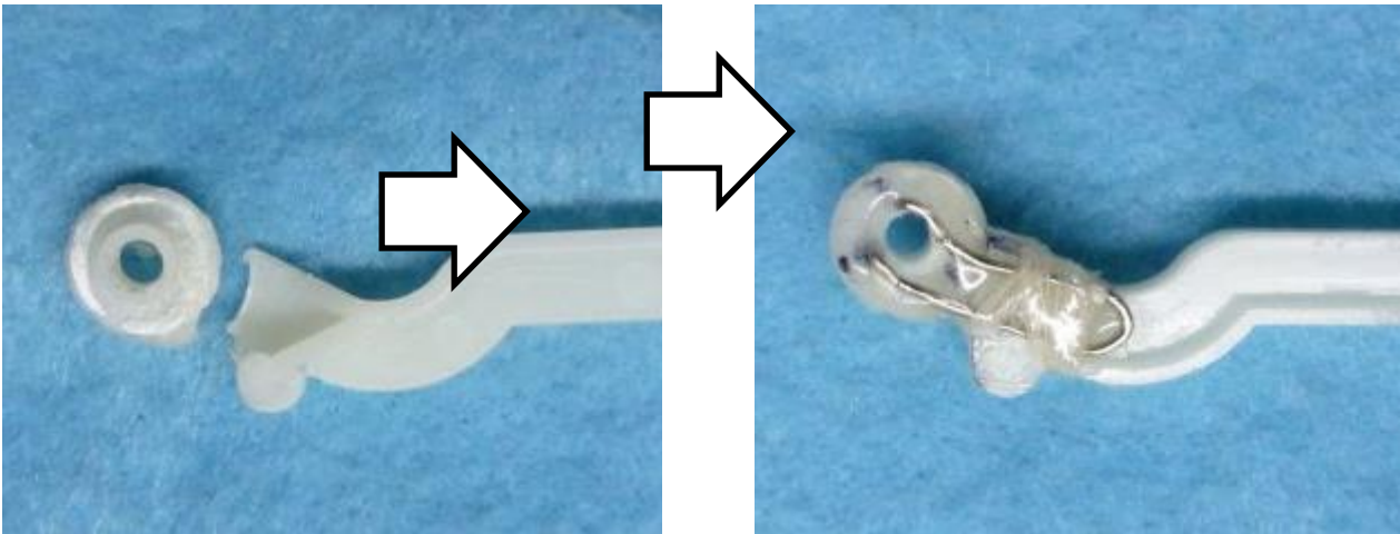
例4 修復前 ⇒ ステンレス線φ0.3+φ0.9+縫製糸+エポキシ接着剤
