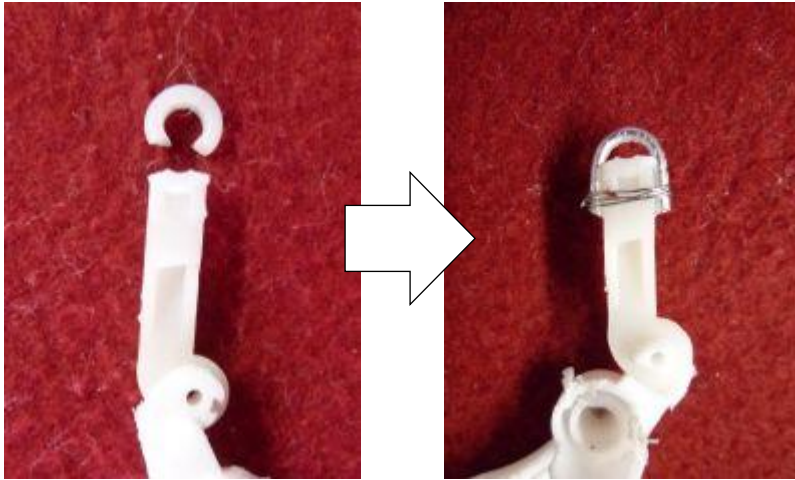
例2 修復前 ⇒ ステンレス線φ0.3+アルミ線φ0.9+PPX
