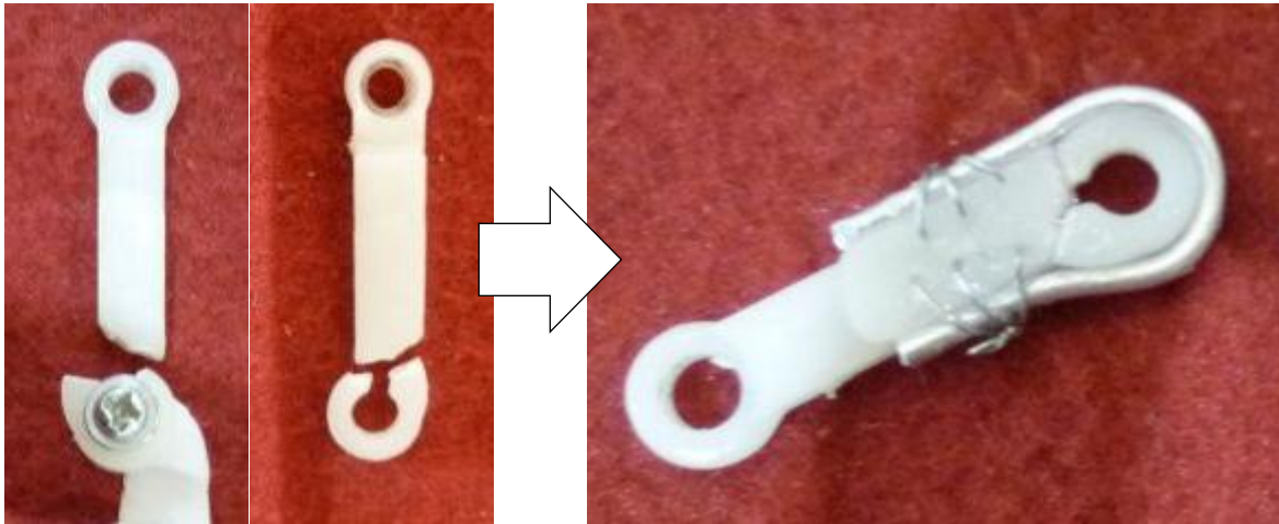
例3 修復前 ⇒ ステンレス線φ0.3+アルミ線φ0.9+PPX
