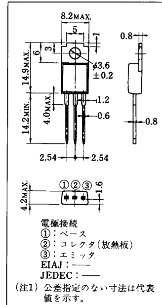
外形図
